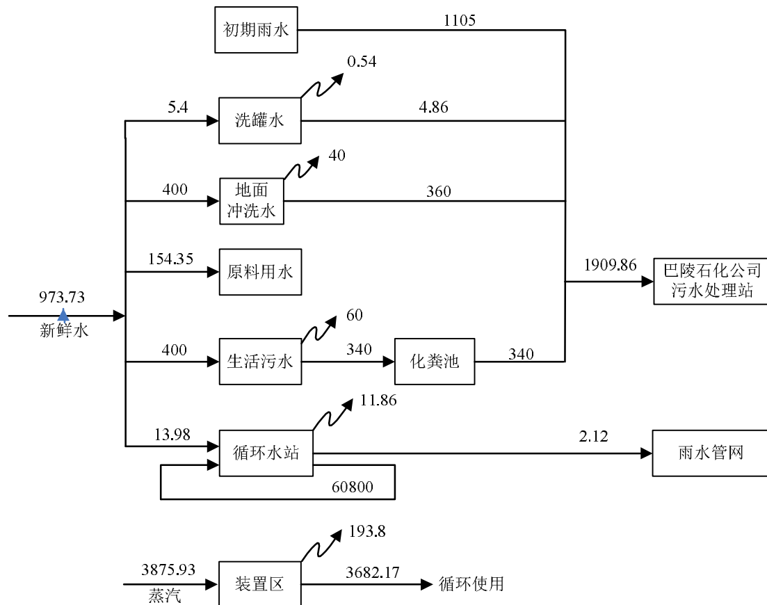
图 3-20 项目水平衡图 (单位 \text{m}^3/\text{a} )
