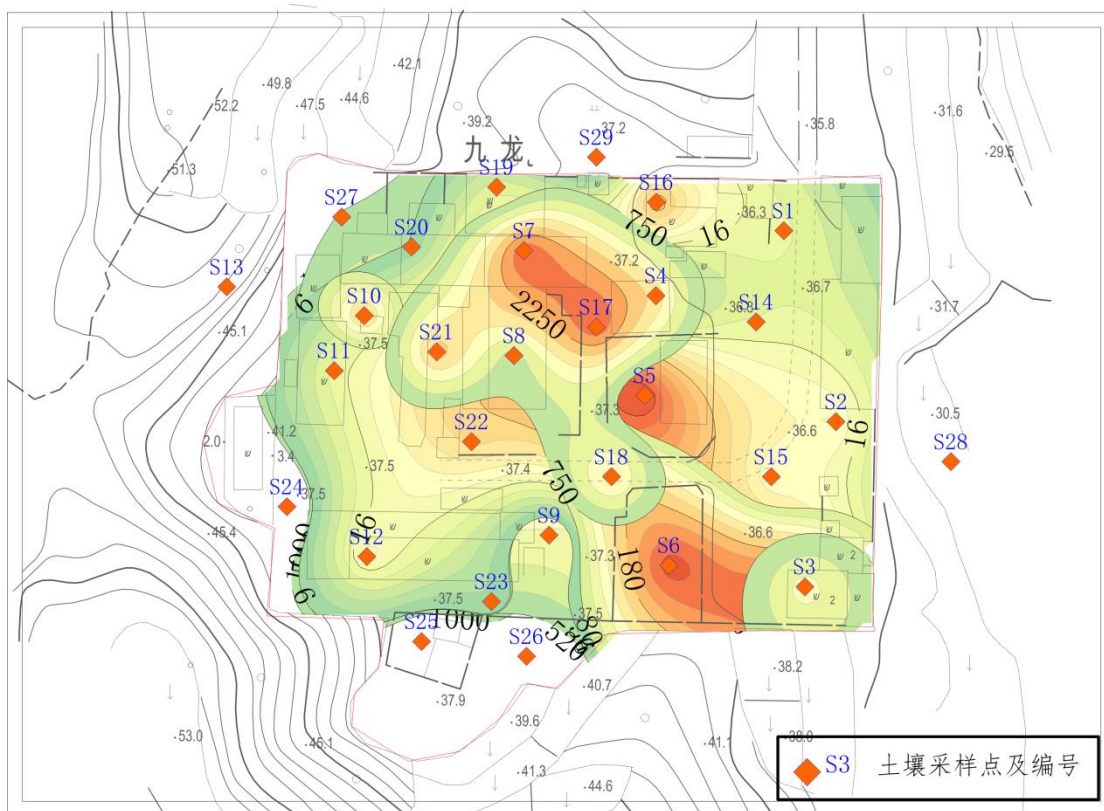
图 3.6-1 0-2m 深度内土壤修复范围
