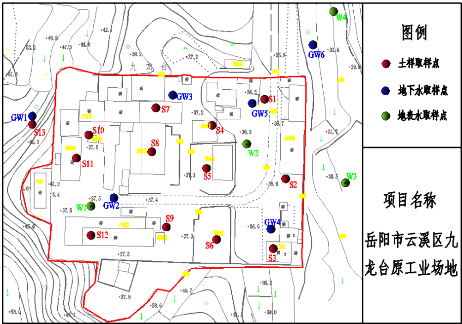
图 3.5-2 场地初步调查采样点布设
