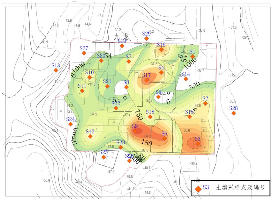
图 3.6-2 2-4m 深度内土壤修复范围
