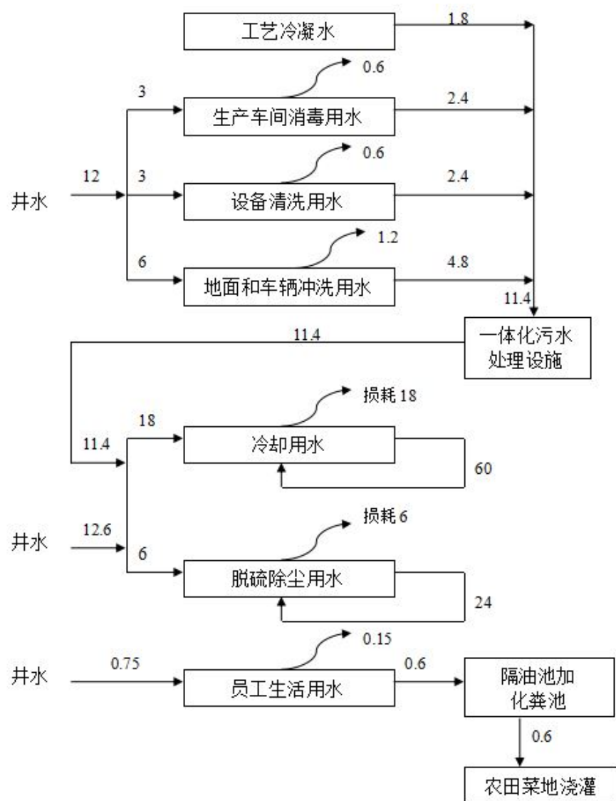
图 3 水量平衡图 ( \text{m}^3/\text{d} )
