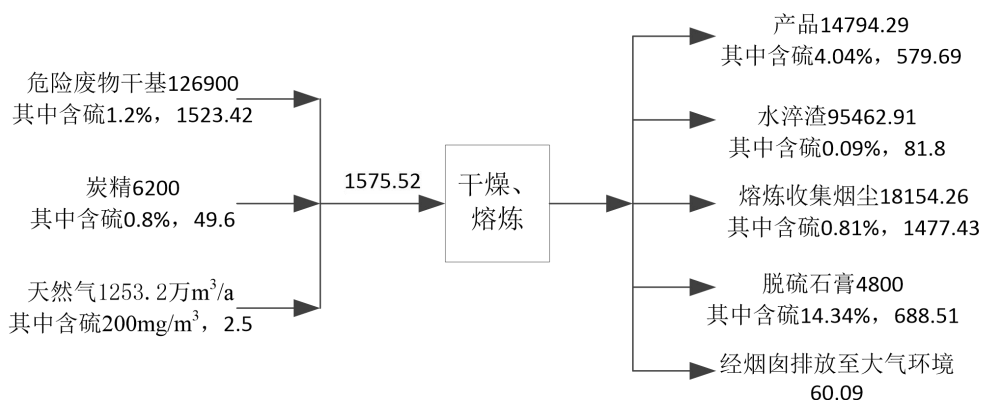
图 2.2-12 硫元素平衡图 单位：t/a
