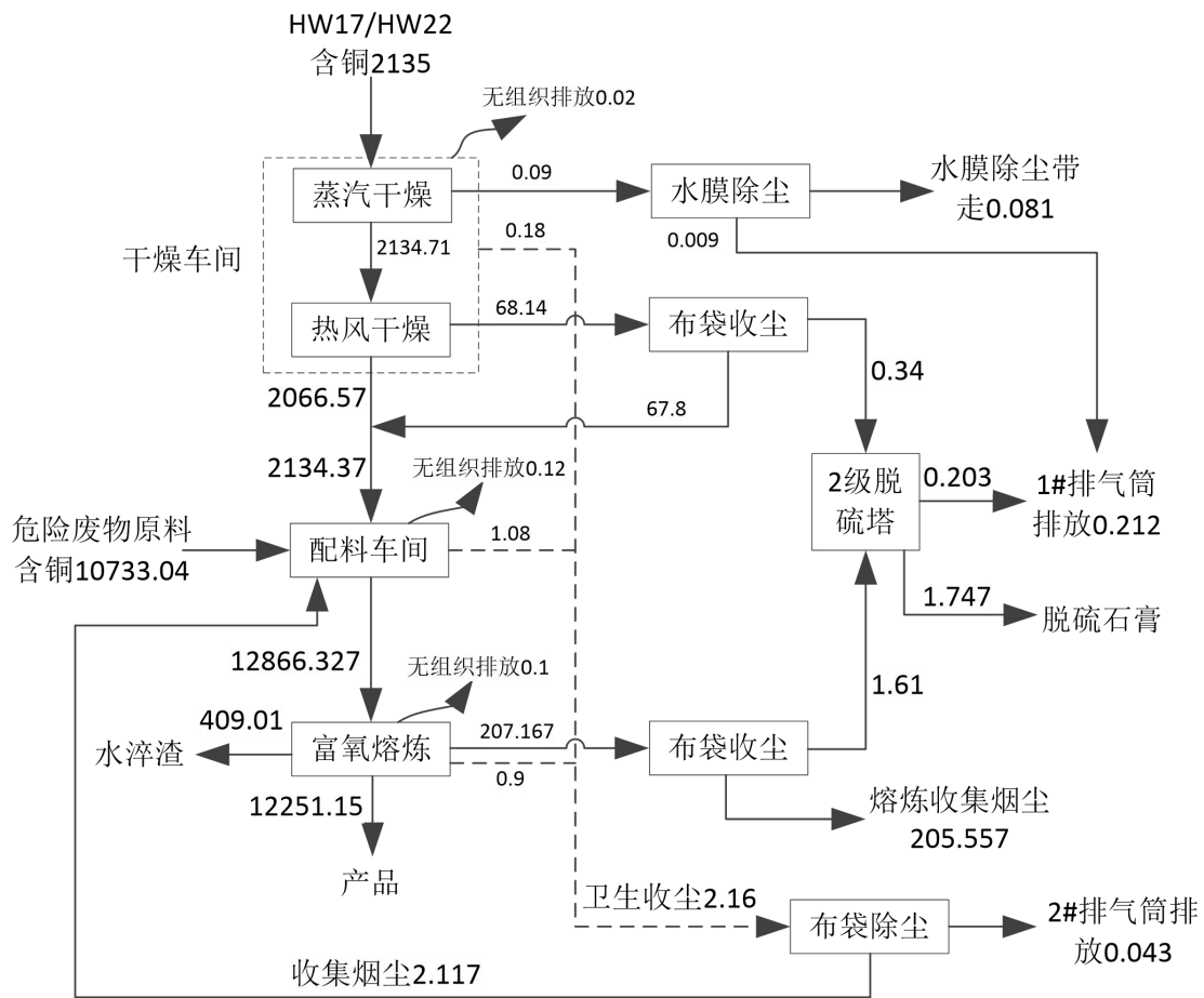
图 2.2-2 铜元素平衡图 单位: t/a
