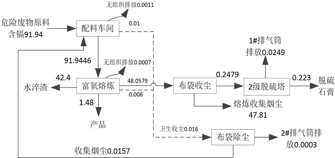
图 2.2-8 镉元素平衡表 单位：t/a
