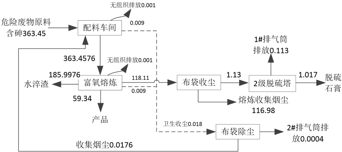
图 2.2-6 砷元素平衡表 单位：t/a
