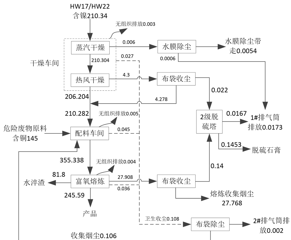
图 2.2-3 镍元素平衡图 单位: t/a
