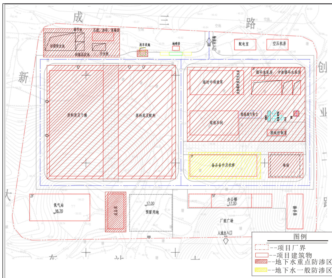
图 7.6-1 项目地下水分区防渗图
