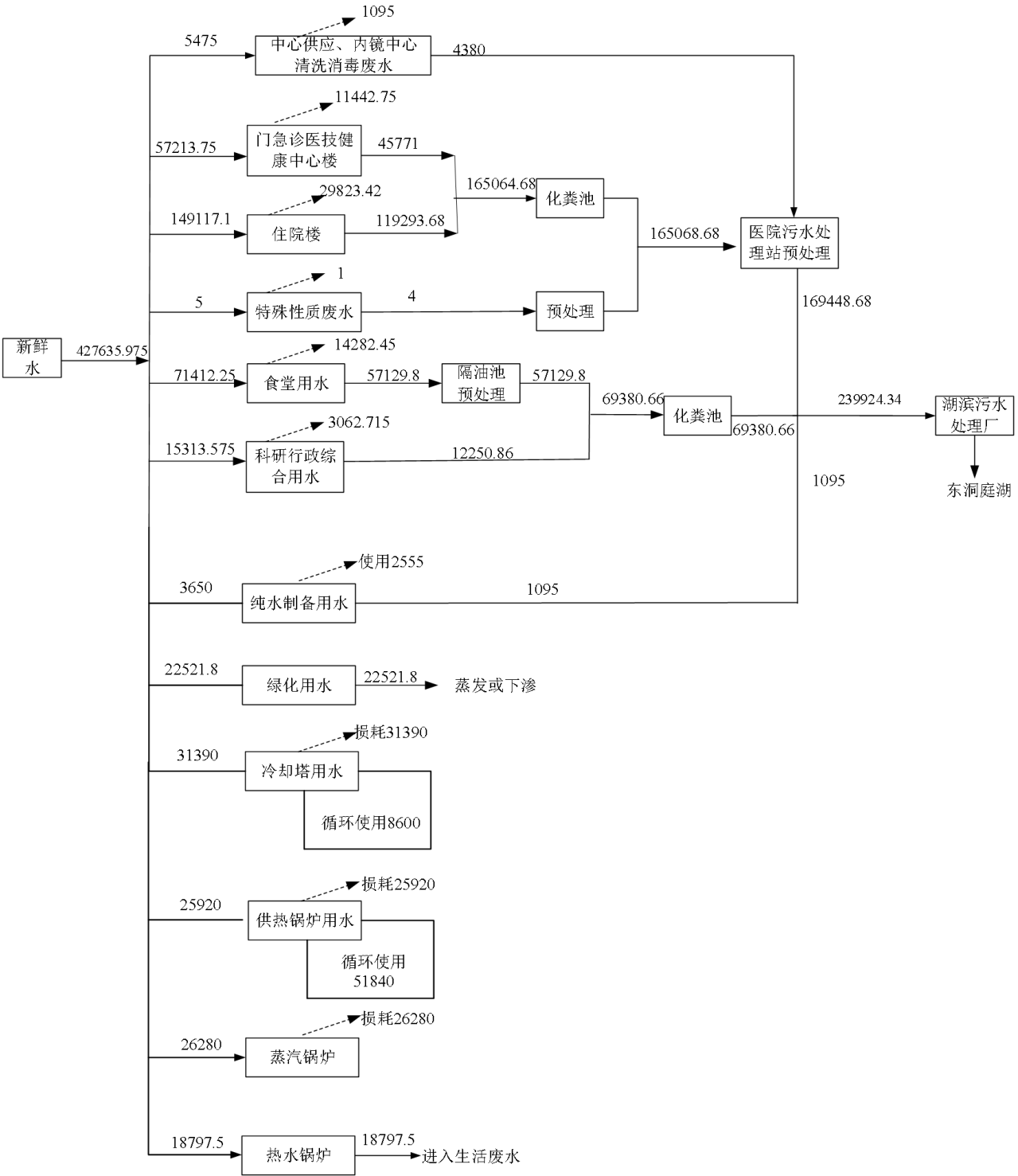
图 3.3-2 项目年水平衡图 (m³/a)
