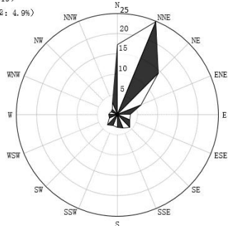
累年3月风向频率统计图
