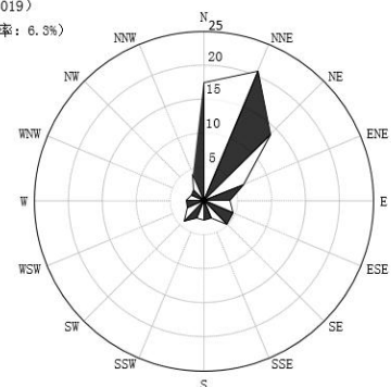
图 6.1-2 岳阳气象站月风向玫瑰图
