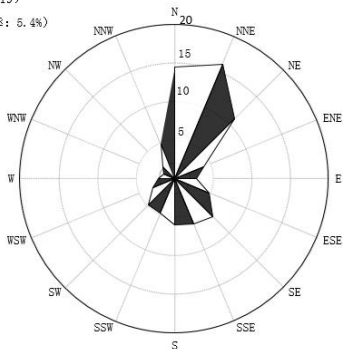
累年5月风向频率统计图
