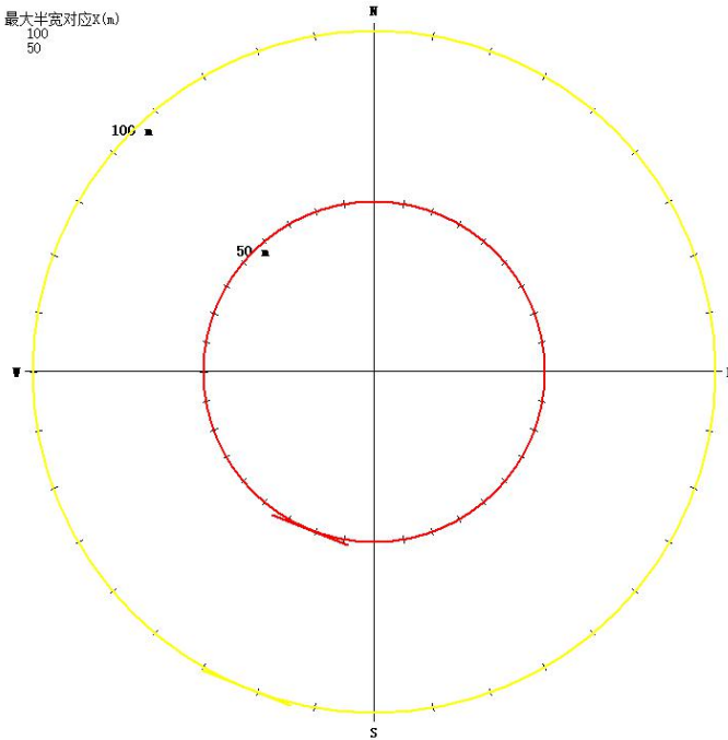
图 8.8-8b 四甲基氯硅烷达到不同毒性终点浓度的最大影响范围（最常见气象条件）
