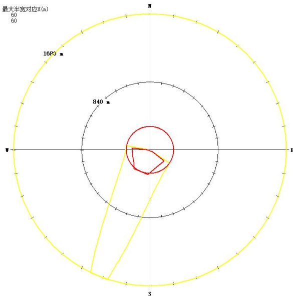
图 8.8-2a 甲基二氯硅烷预测浓度达到不同毒性终点浓度的最大影响范围 (最不利气象条件)
