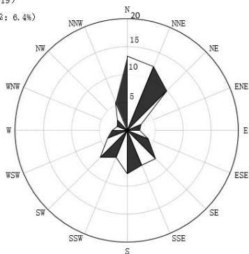
累年5月风向频率统计图
