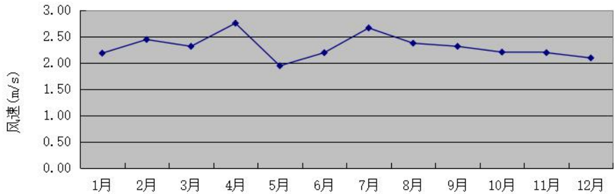
图 6.1-6 2019 年年平均风速月变化曲线
