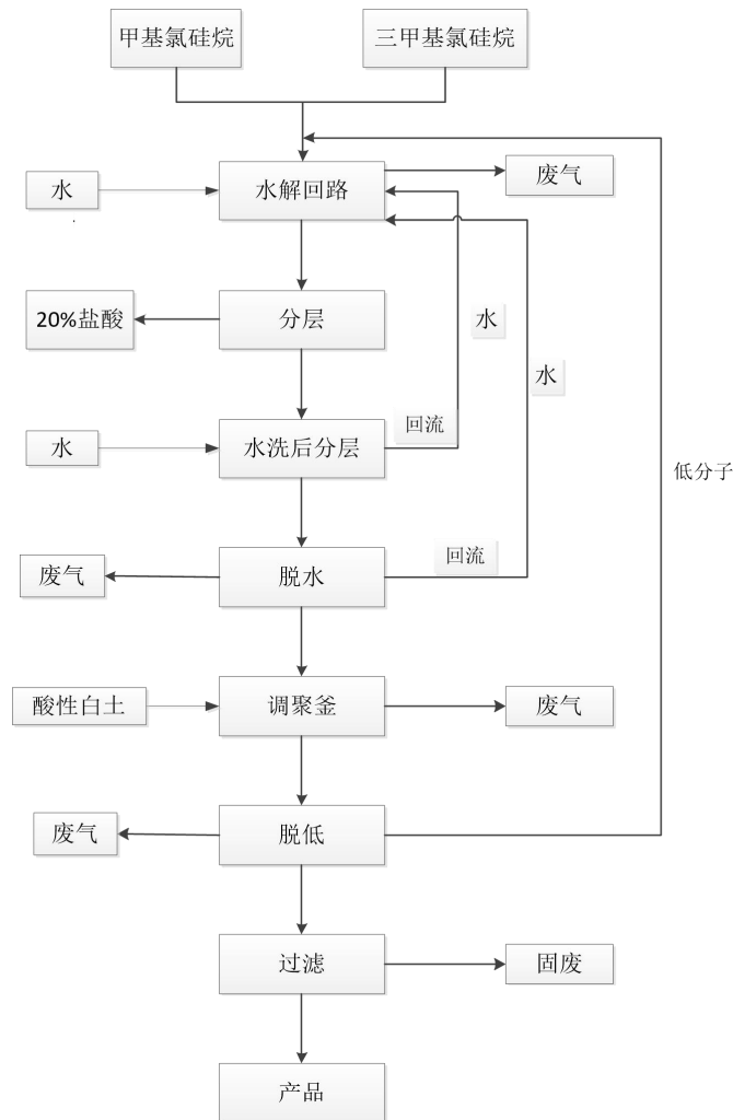
图 4.3-1 本项目功能性硅油生产工艺流程和产污环节示意图
