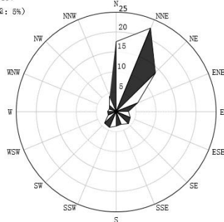
累年2月风向频率统计图
