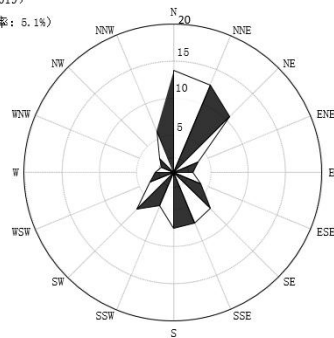
累年4月风向频率统计图
