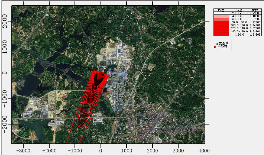
图 8.8-1a 甲基二氯硅烷预测浓度范围分布图（最不利气象条件）
