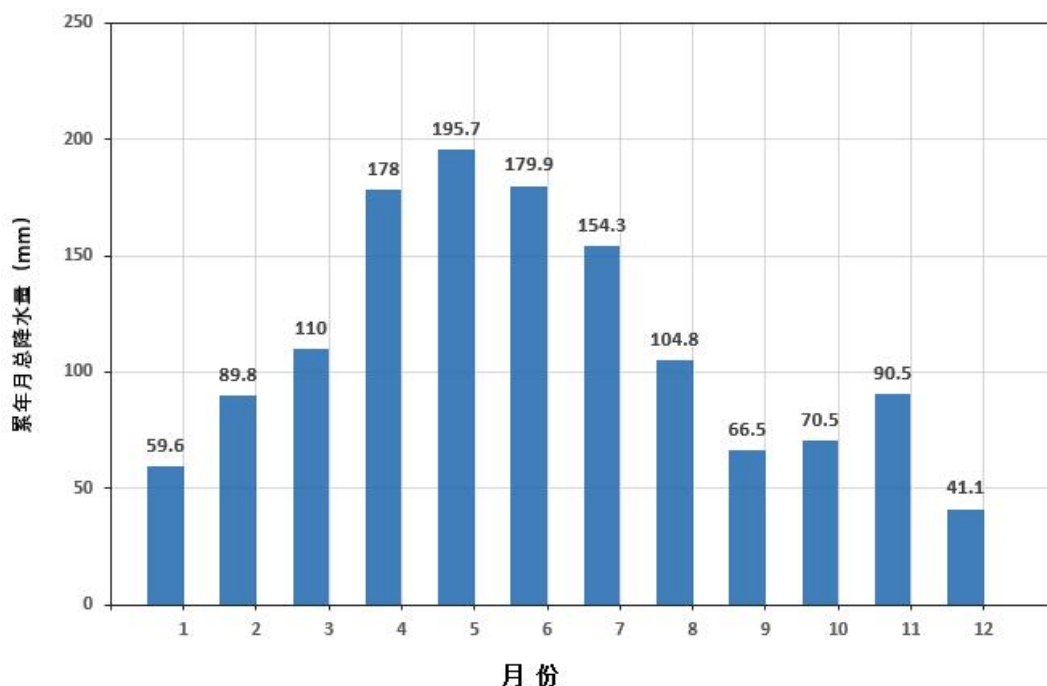
图 6.1-4 岳阳累年月平均降水量 (单位: 毫米)
