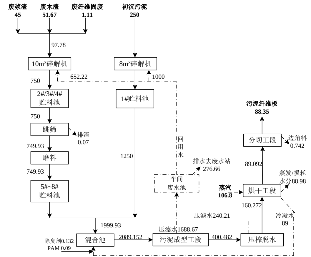
图 2-2 项目物料平衡走向流程图 单位 t/d
