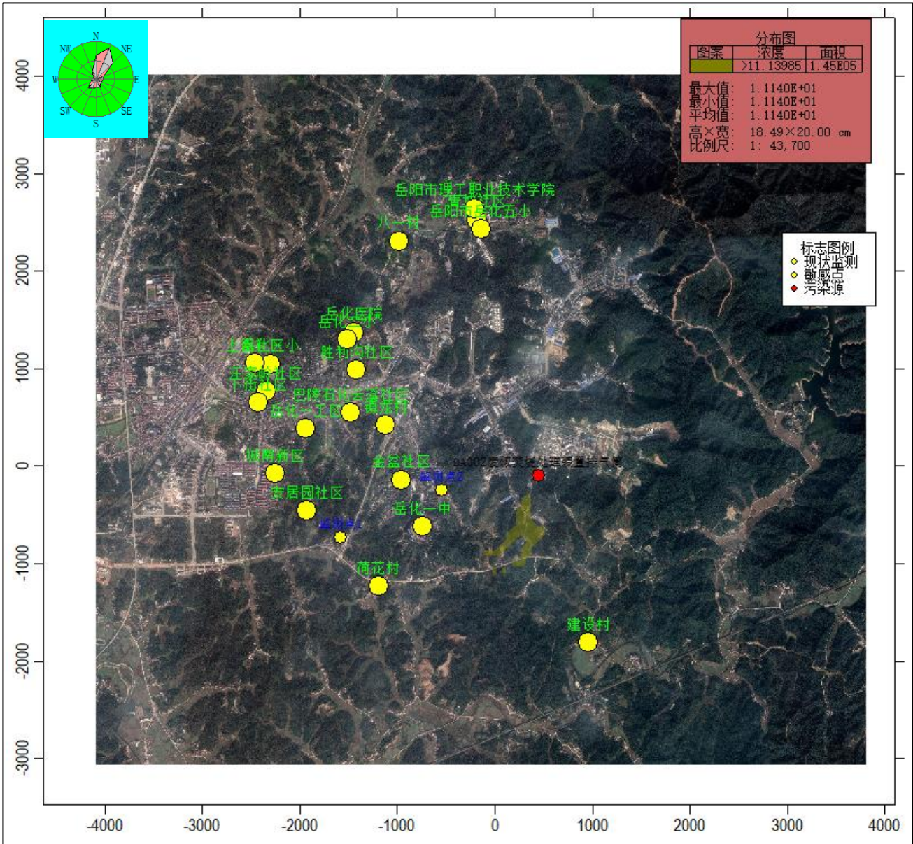
图6.2-12 PM 2.5 叠加后最大年平均浓度分布图（单位：μg/m 3 ）
