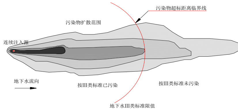
图6.2-17 一维稳定流动一维水动力弥散问题污染物运移示意图
