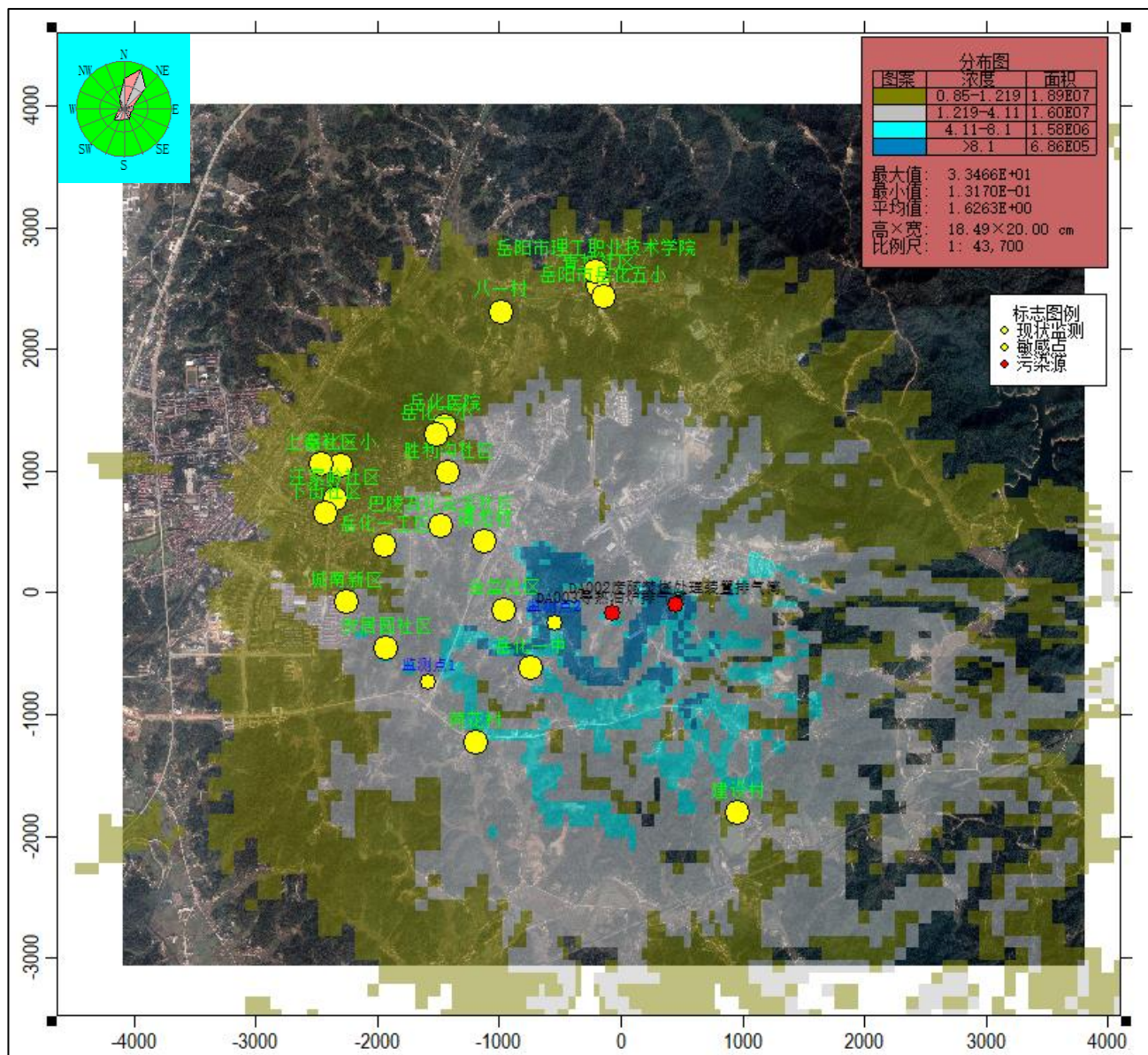
图6.2-7 NO 2 叠加后最大小时平均浓度分布图 (单位: \mu\text{g}/\text{m}^3 )
