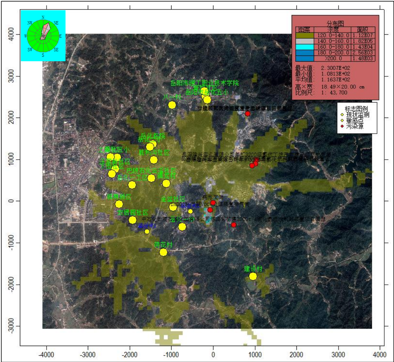
图6.2-3 VOCs 叠加后最大日平均浓度分布图（单位：μg/m³）
