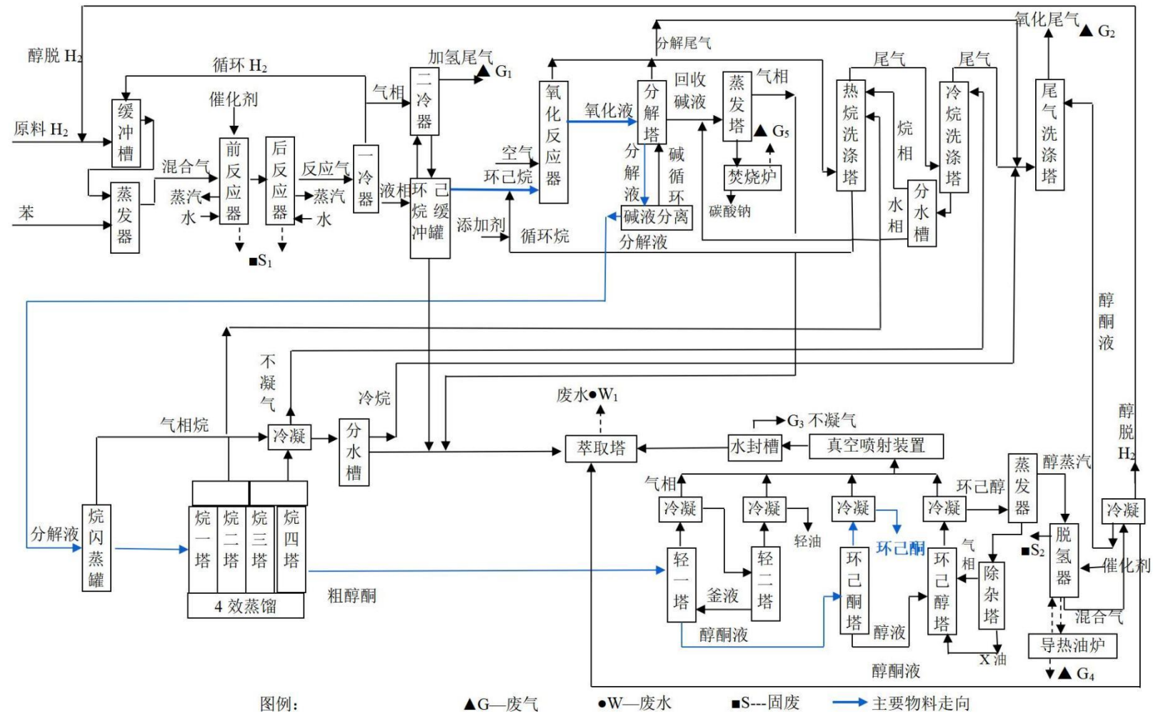
图3.8-1 现有工艺流程及产污环节图
