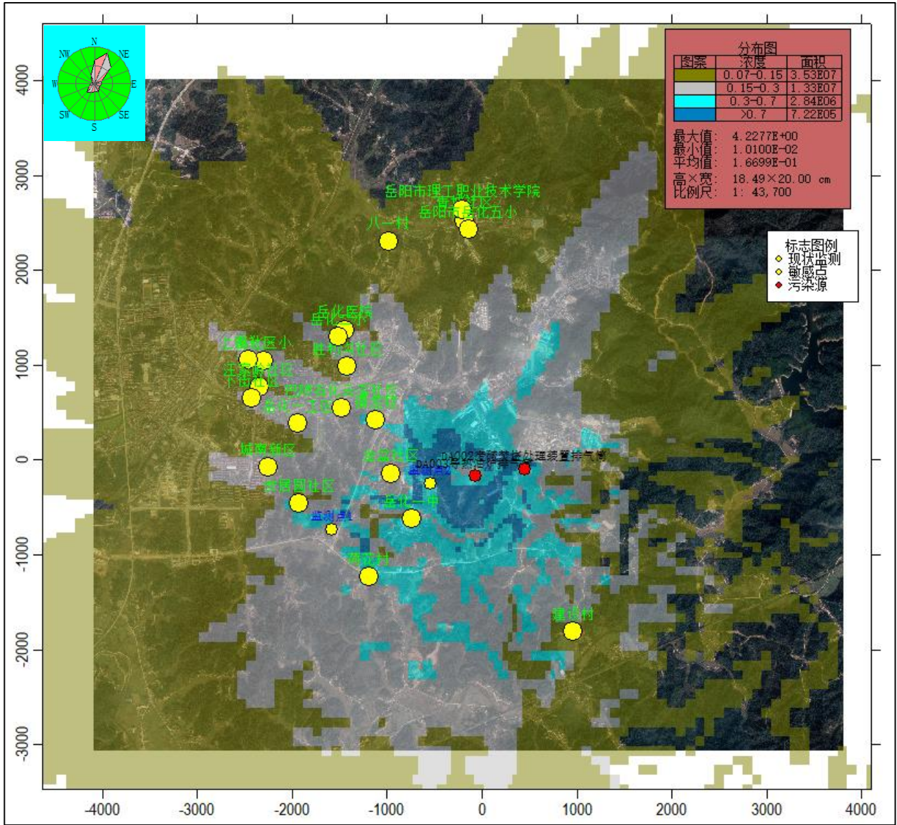
图6.2-8 NO 2 叠加后最大日平均浓度分布图（单位：μg/m 3 ）
