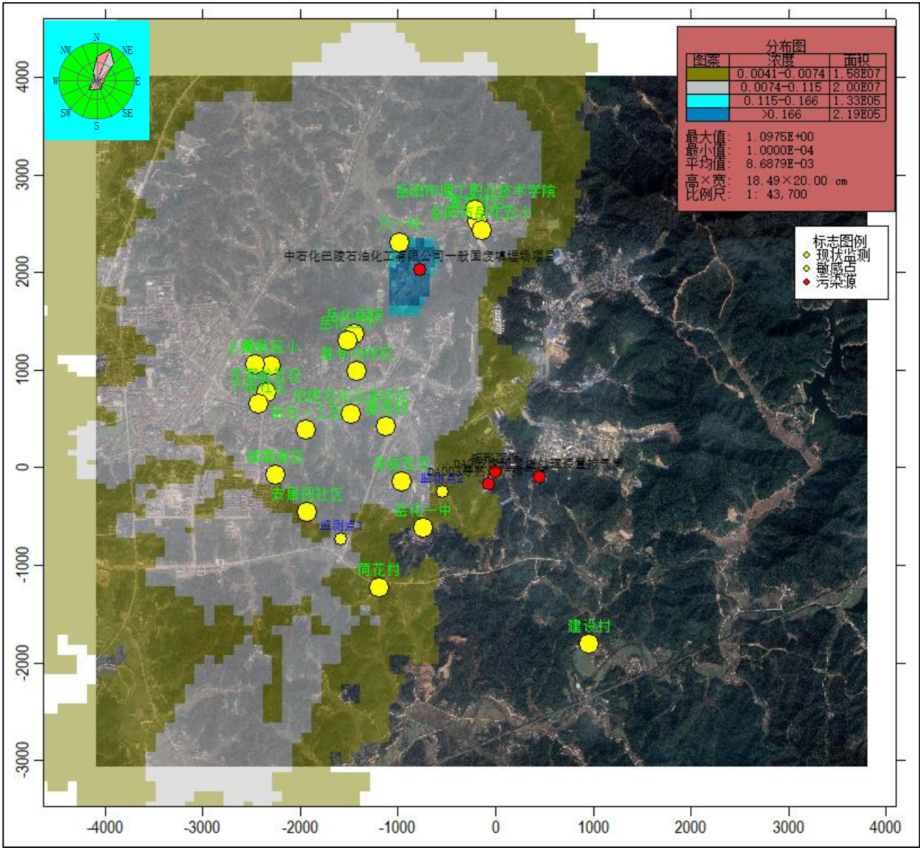
图6.2-2 TSP 叠加后最大年平均浓度分布图（单位：μg/m 3 ）
