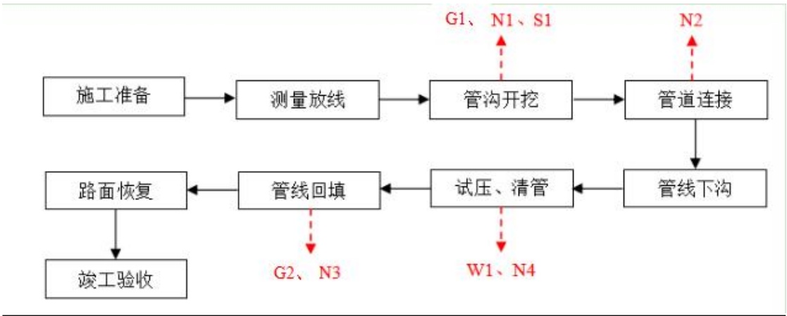
图 2-1 本项目管线施工工艺流程及产排污环节图 新建雨污管道施工工艺流程简述：
