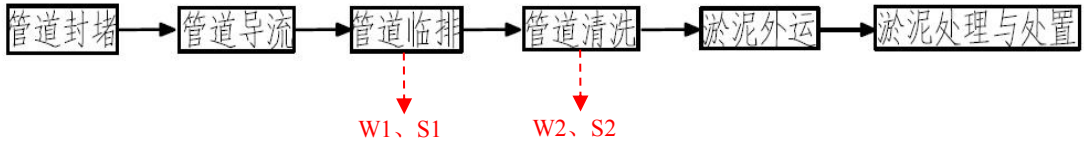
图 2-3 本项目清淤施工工艺流程图
