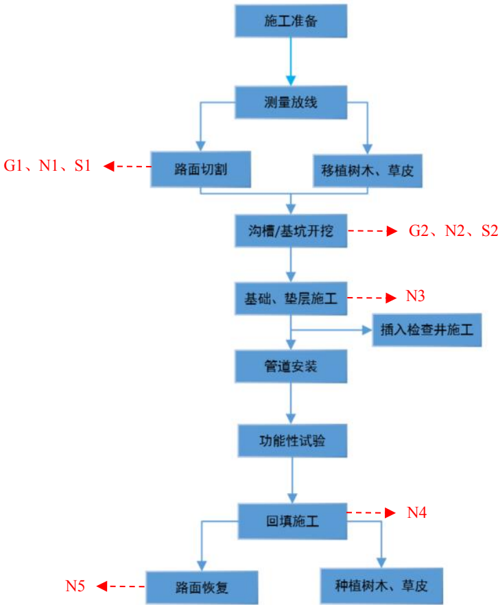
图 2-4 本项目开挖修复施工工艺流程图
