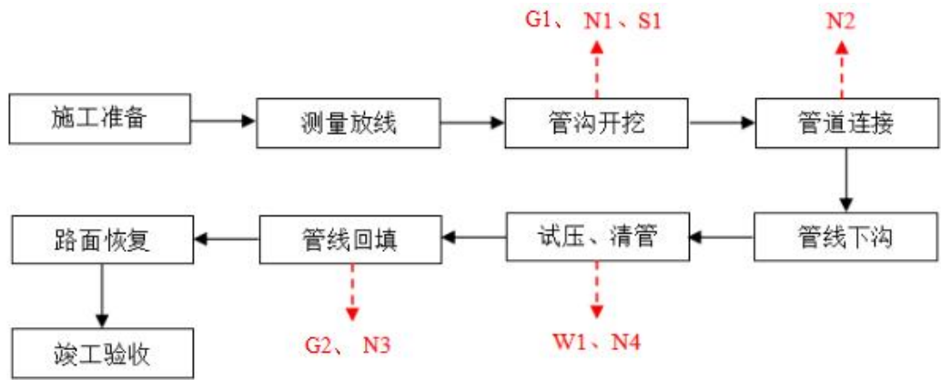
图 2-1 本项目新建雨污管道施工工艺流程及产排污环节图 新建雨污管道施工工艺流程简述：
