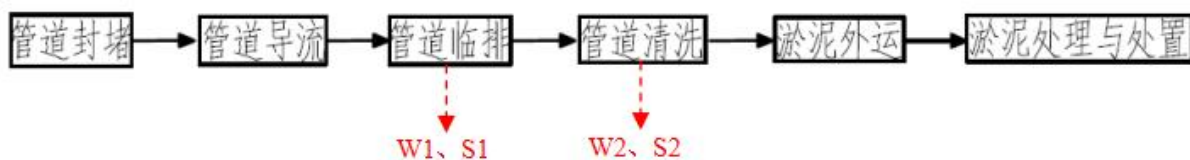
图 2-3 本项目清淤施工工艺流程图
