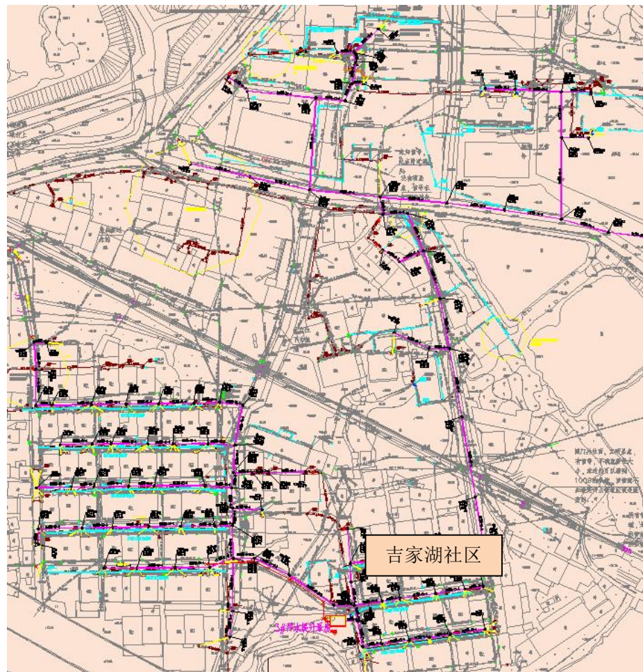
附图 3-5 2#泵站、3#泵站平面布置及周边环境示意图
