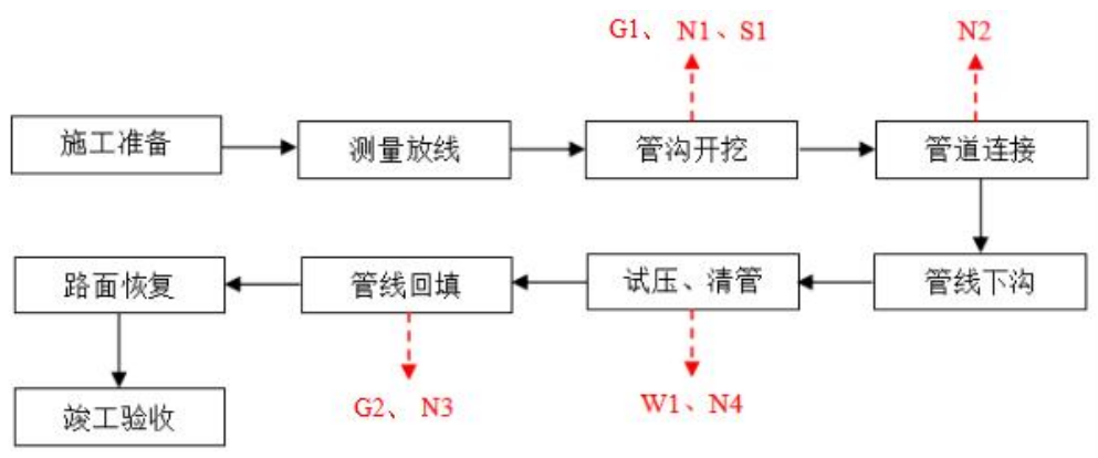
图 2-1 本项目新建雨污管道施工工艺流程及产排污环节图
