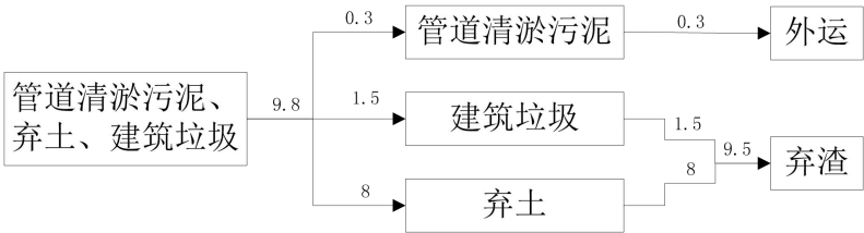
图 4-1 土石方平衡图 单位：万 m 3
