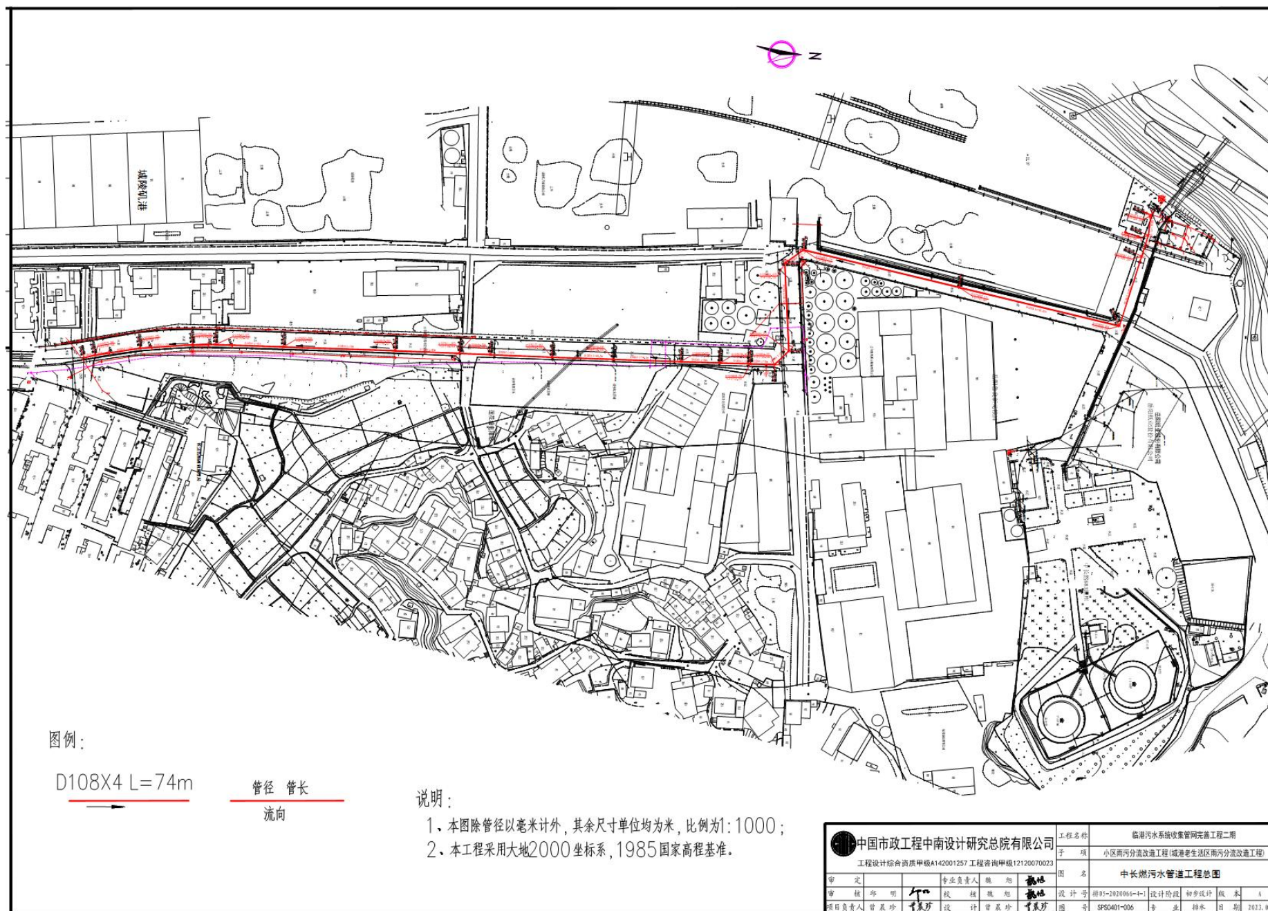
附图 3-2 中长燃污水管道工程平面布置图
