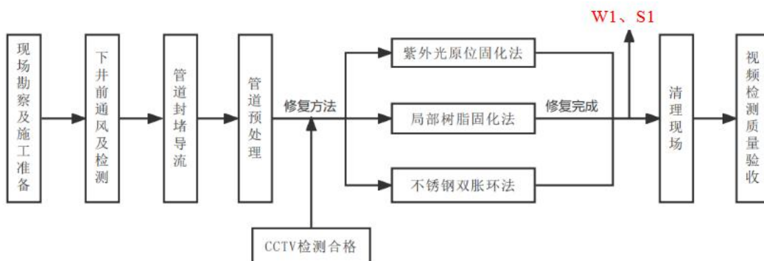
图 2-4 本项目开挖修复施工工艺流程图
