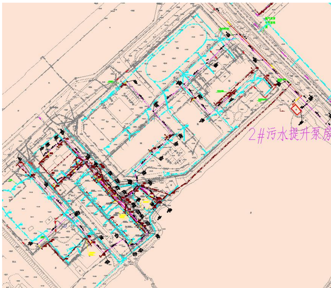
附图 3-5 2#泵站、3#泵站平面布置及周边环境示意图
