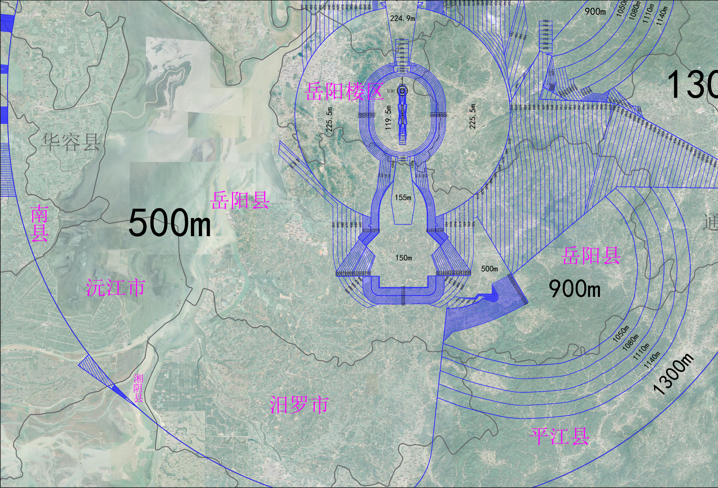
附图04：岳阳三荷机场航行服务程序净空保护区域一体化图（岳阳县、岳阳楼区、南县、沅江市、湘阴县、汨罗市、平江县分图） 比例尺：1:25万
