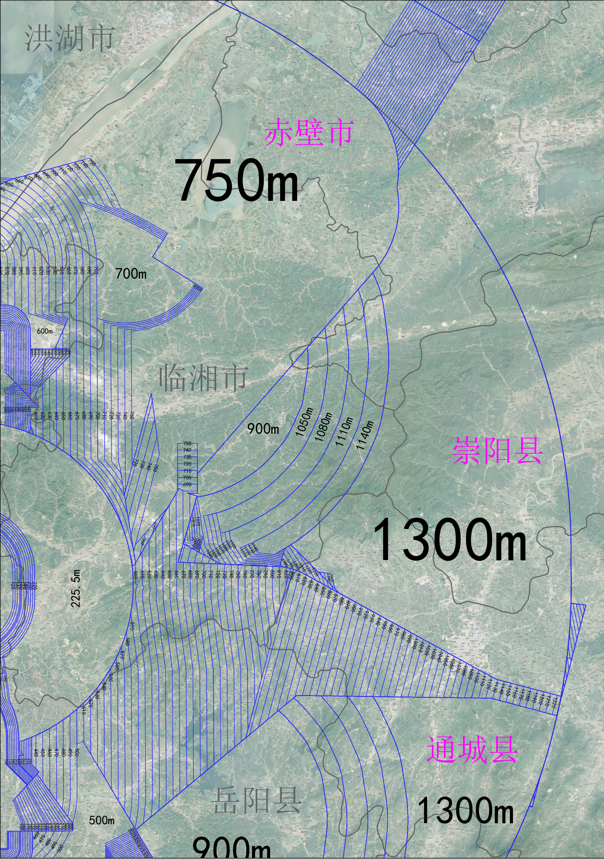
附图06：岳阳三荷机场航行服务程序净空保护区域一体化图（赤壁市、崇阳县、通城县分图）比例尺：1:20万
