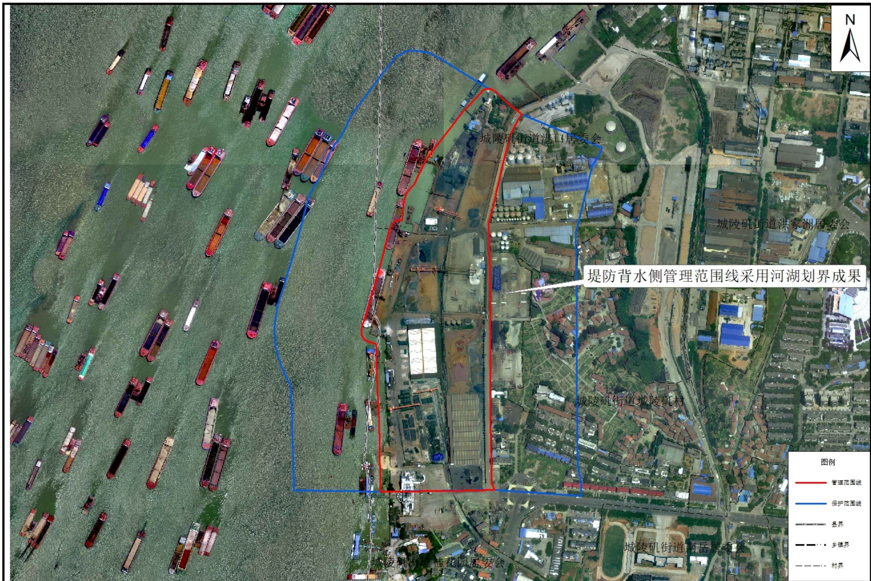
长江干堤城陵矶段管理与保护范围划界成果示意图
