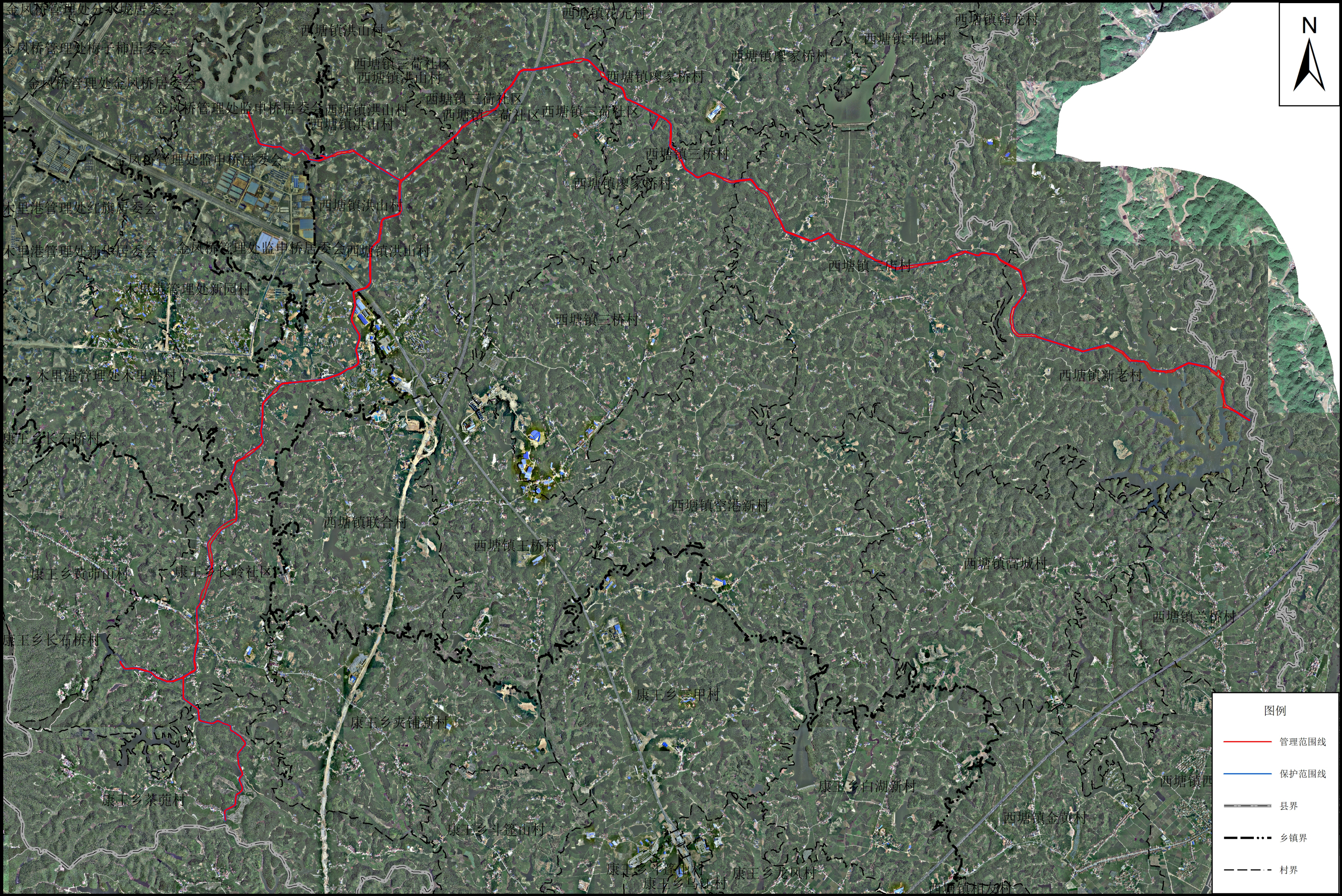
铁山灌区管理与保护范围划界成果示意图（岳阳楼区部分）
