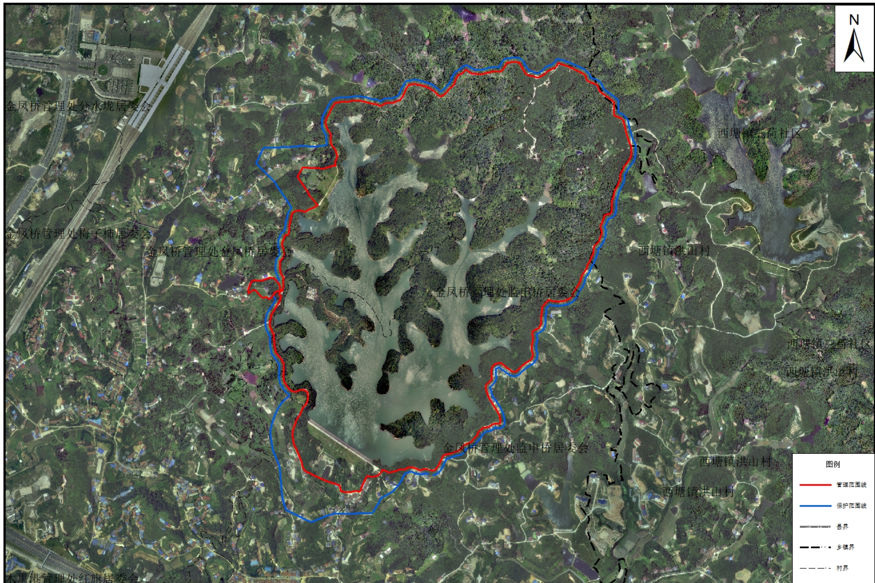
金凤水库管理与保护范围划界成果示意图
