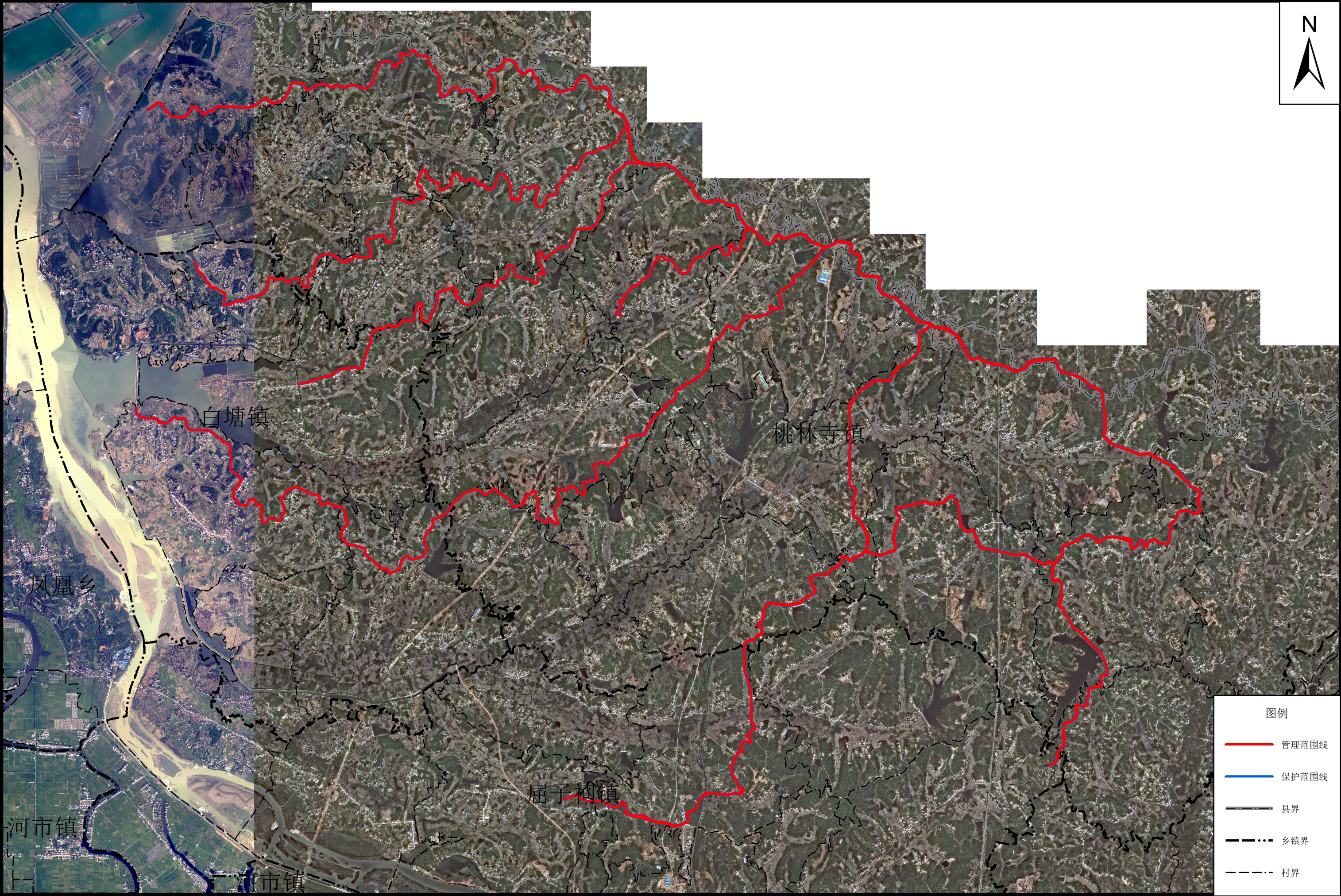
铁山灌区管理与保护范围划界成果示意图(汨罗市部分)
