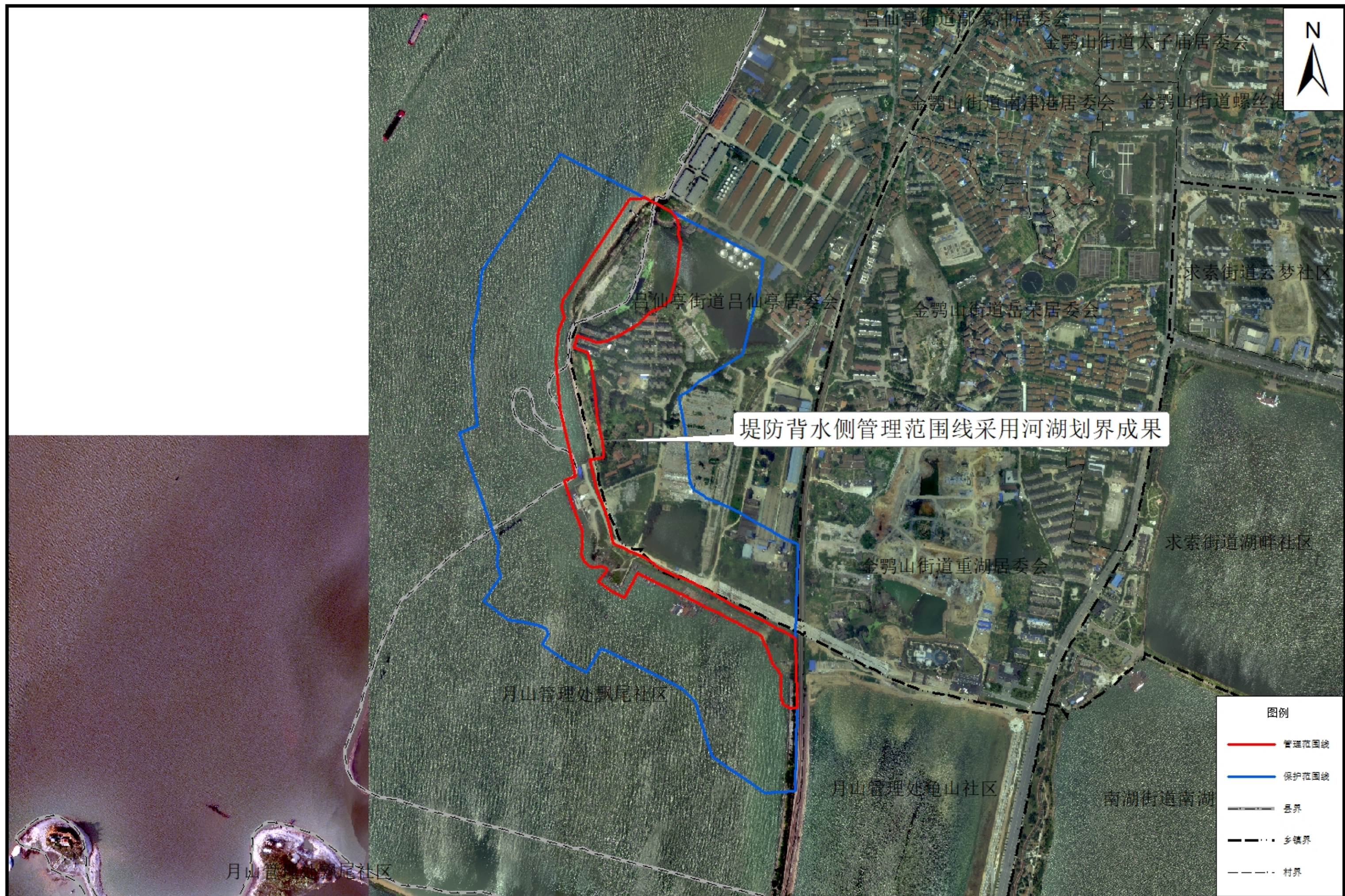
韩家湾大堤管理与保护范围划界成果示意图
