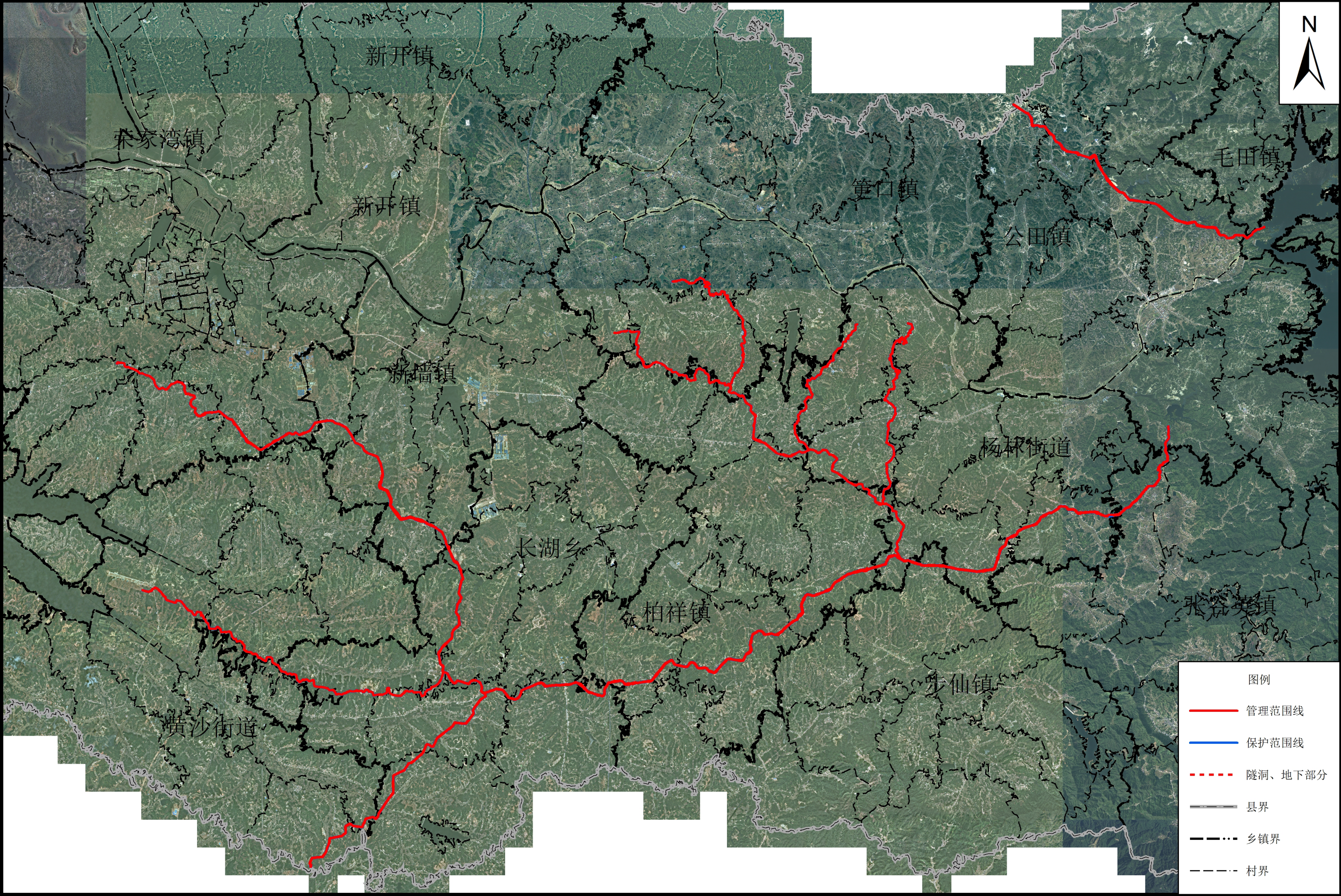
铁山灌区管理与保护范围划界成果示意图（岳阳县部分）
