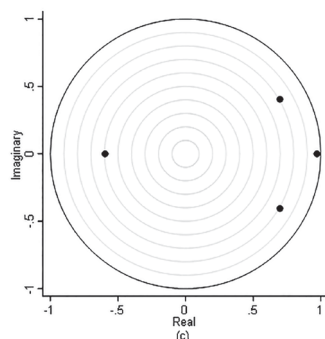
图1 VAR系统的稳定性检验
