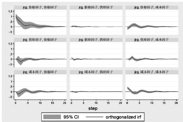
图1 正交化的脉冲响应
